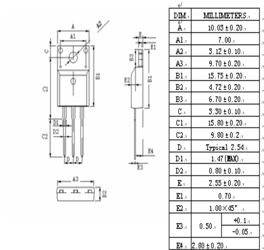
TO-220F 外形尺寸图
